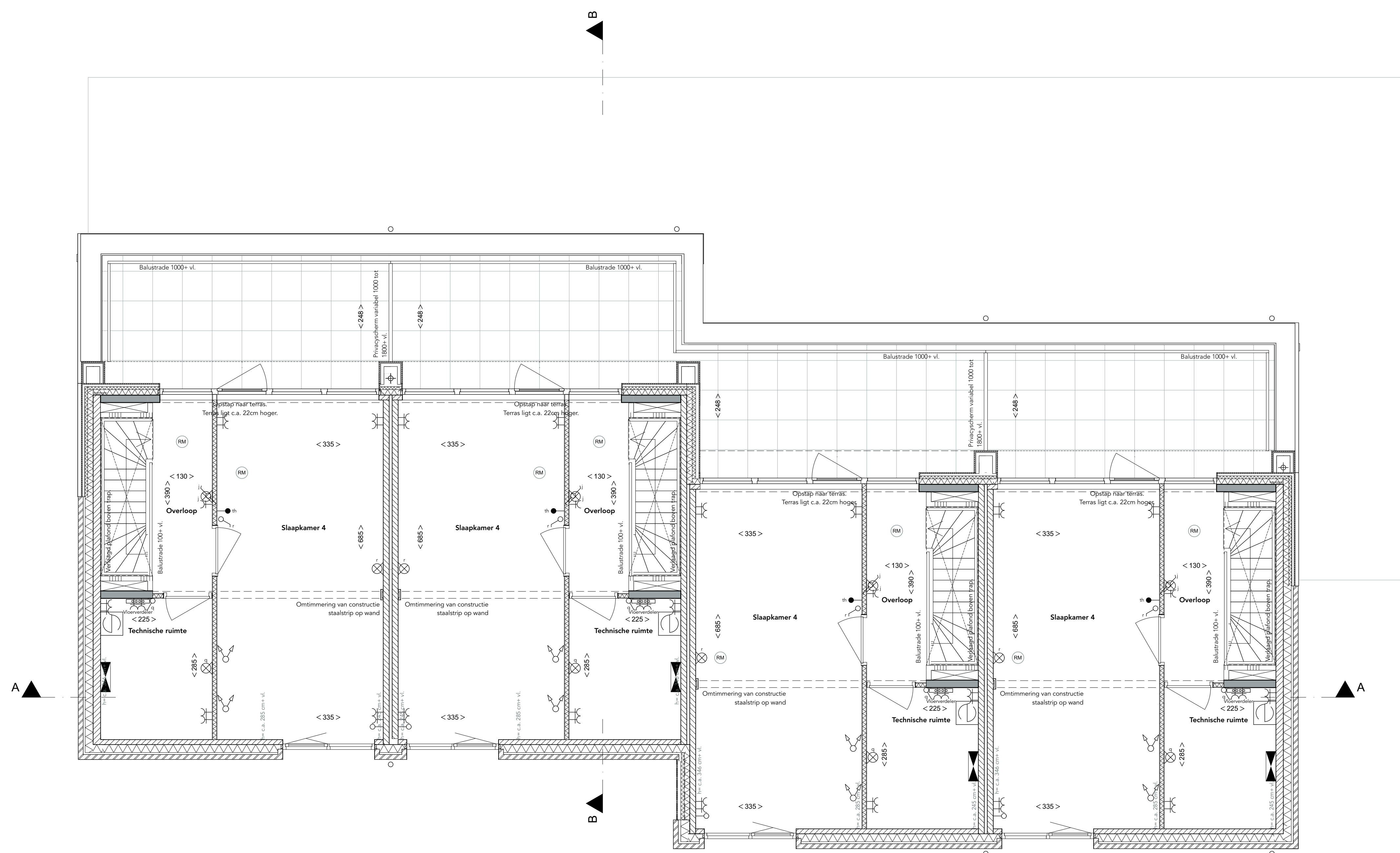
3e verdieping Schaal 1:50
